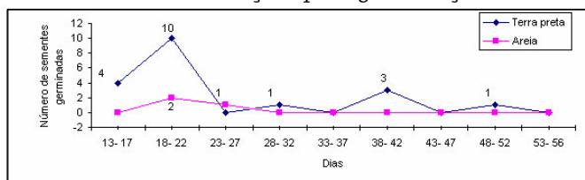
FIG. 1 - Número de sementes germinadas de Cedrela odorata L. por propagação sexuada após 56 dias de germinação das sementes em terra preta e areia.
