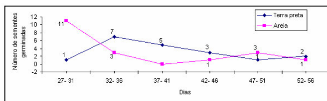
FIG. 3 - Número de sementes germinadas Virola surinamensis (Rol. ex Rottb) Warb. por propagação sexuada após 56 dias de germinação das sementes em terra preta e areia.
