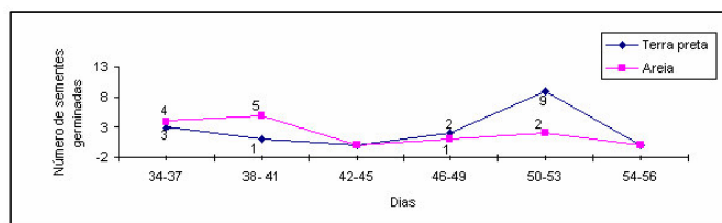
FIG. 2 - Número de sementes germinadas de Licaria mahuba (A. Samp.) Kosterm. por propagação sexuada após 56 dias de germinação das sementes em terra preta e areia.
