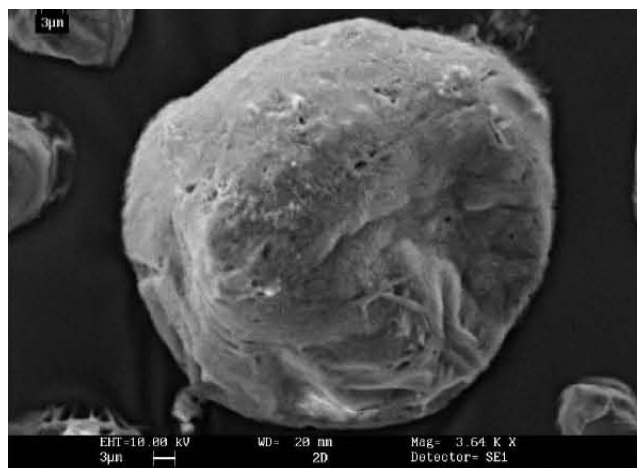
FIG. 2 - Micrografias obtidas através de microscopia eletrônica de varredura de nanopartícula de quitosana reticulada com tripolifosfato (Silva, 2006).
