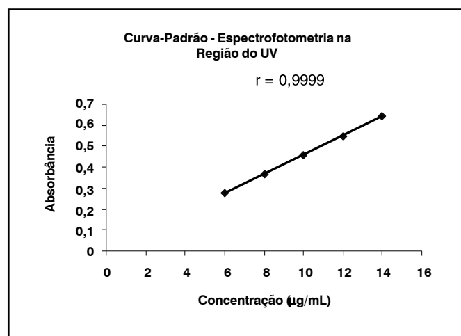
FIG. 2 - Representação gráfica da curva-padrão do piroxicam obtida pelo método espectrofotométrico na região do ultravioleta a 354nm.
