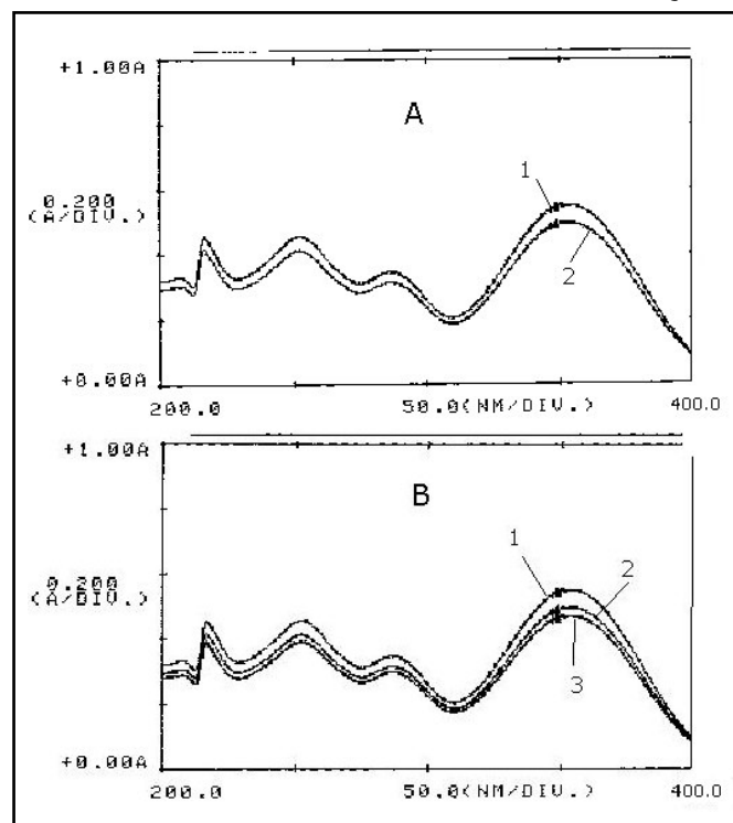
FIG. 1 - Espectro de absorção na região do UV do piroxicam SQR (A1), amostra industrializada (A2), amostra farmácia 1 (B1), amostra farmácia 2 (B2) e amostra farmácia 3 (B3), preparado em hidróxido de sódio 0,1M a concentração de 10 µg/mL.
